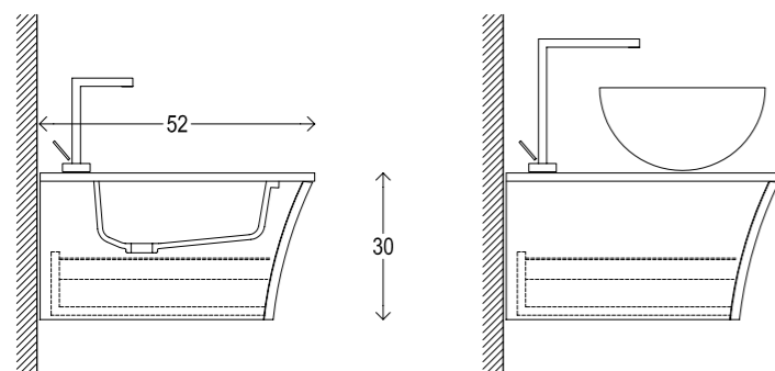
H30DR piano dritto | level plane | plan droite | gerade ebene fläche | encimera recta | ПРЯМАЯ ПАНЕЛЬ
