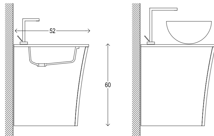
H60DR piano dritto | level plane | plan droite | gerade ebene fläche | encimera recta | ПРЯМАЯ ПАНЕЛЬ
